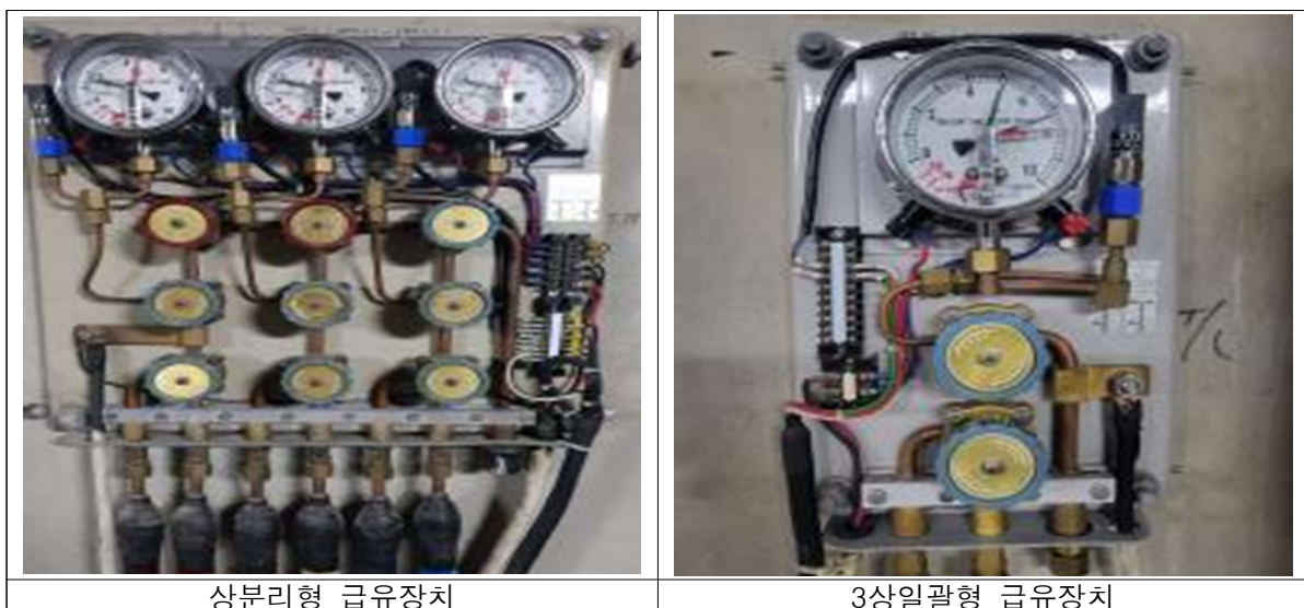
[그림 1] 급유장치의 종류
